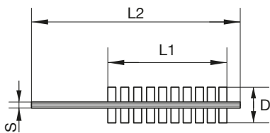
Dimensioni spazzole tubolare
