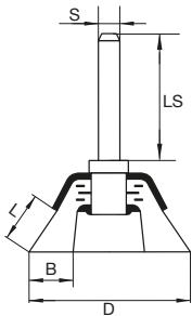
Dimensioni spazzole a tazza con gambo
