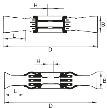
Dimensioni spazzole
