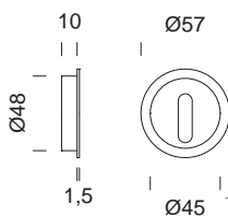
2193/F maniglia incasso foro chiave sliding door handle key hole
