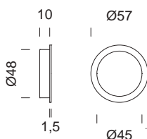
2193 maniglia incasso sliding door handle
